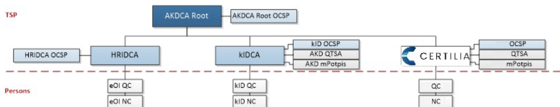
Slika 1: Hijerarhijski model AKD PKI
